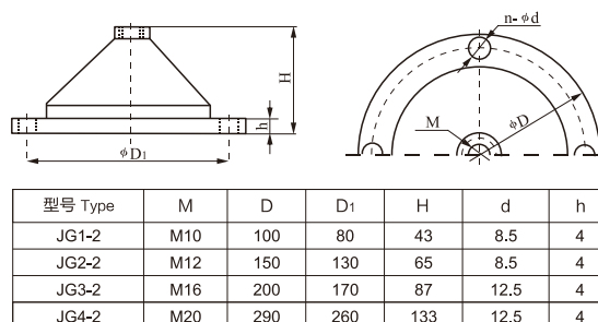
JG型隔振器安装尺寸
